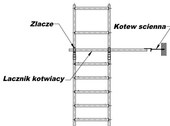
Rys 1. Kotwienie rusztowania
